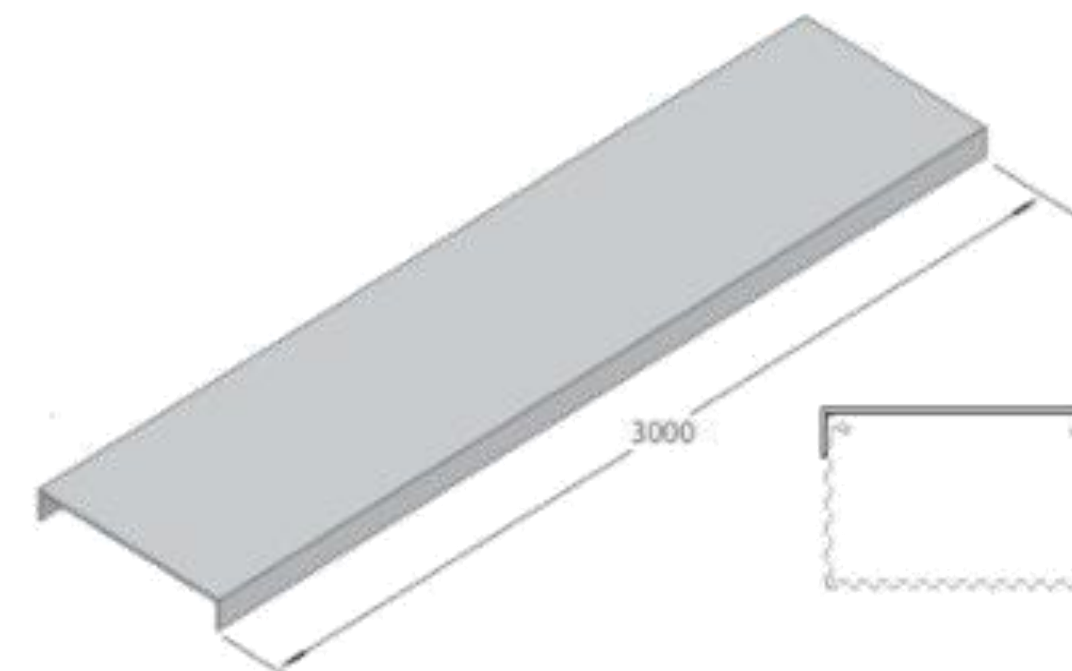
TAMPA DE ENCAIXE – 76 x 3000
