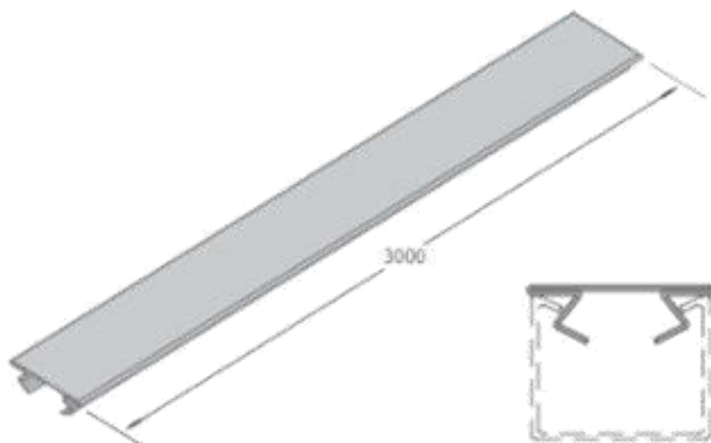
TAMPA DE PRESSÃO – 38 x 3000
