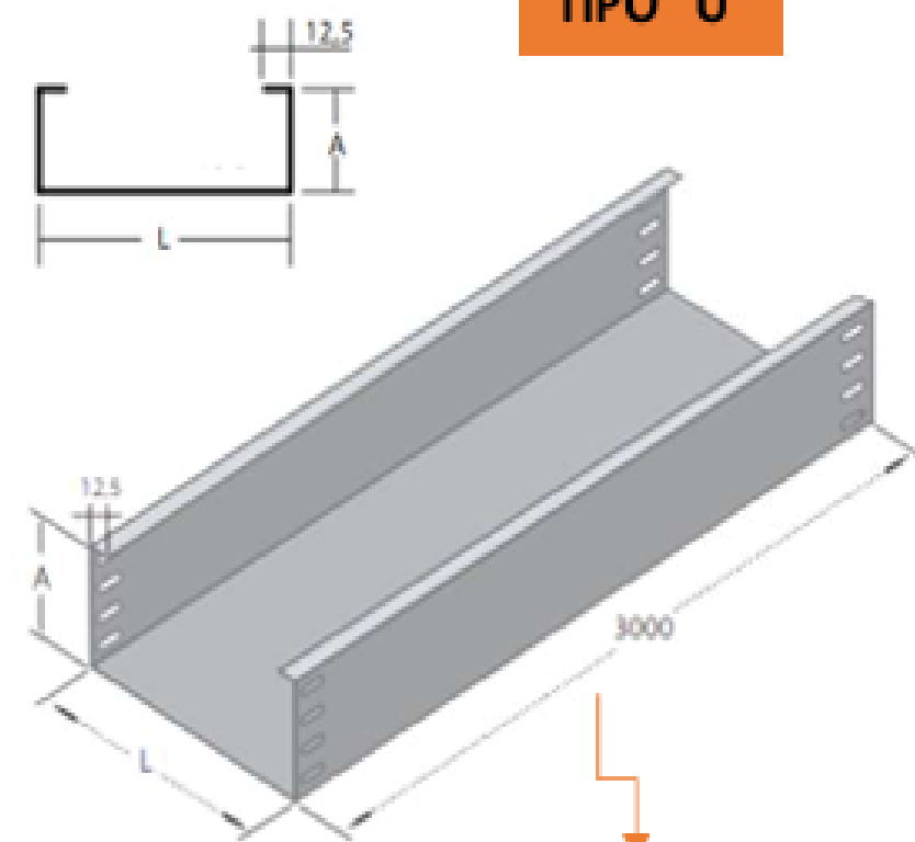
TIPO "U"
