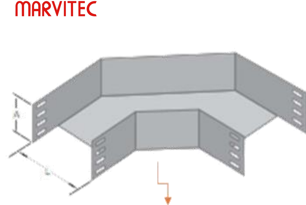
CURVA HORIZONTAL 90°
