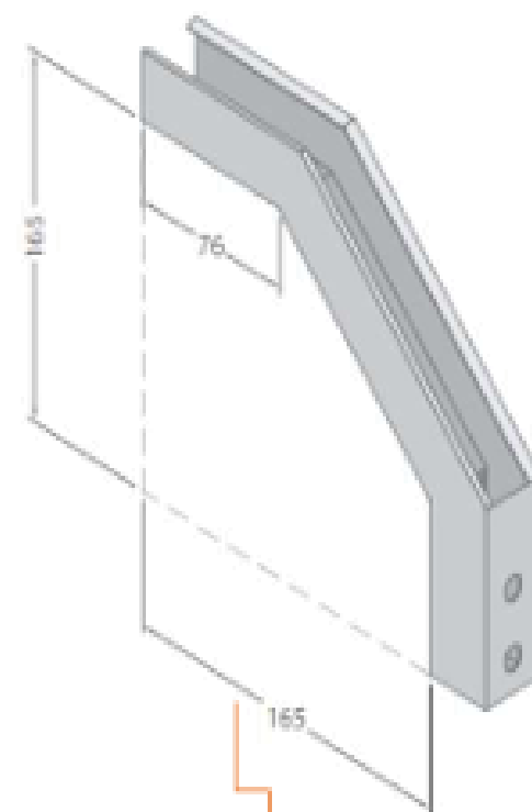
CURVA DE INVERSÃO
