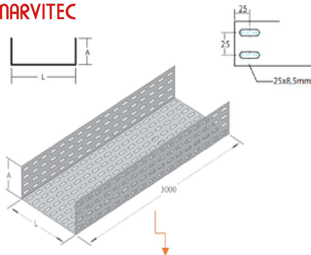
TIPO "U"
