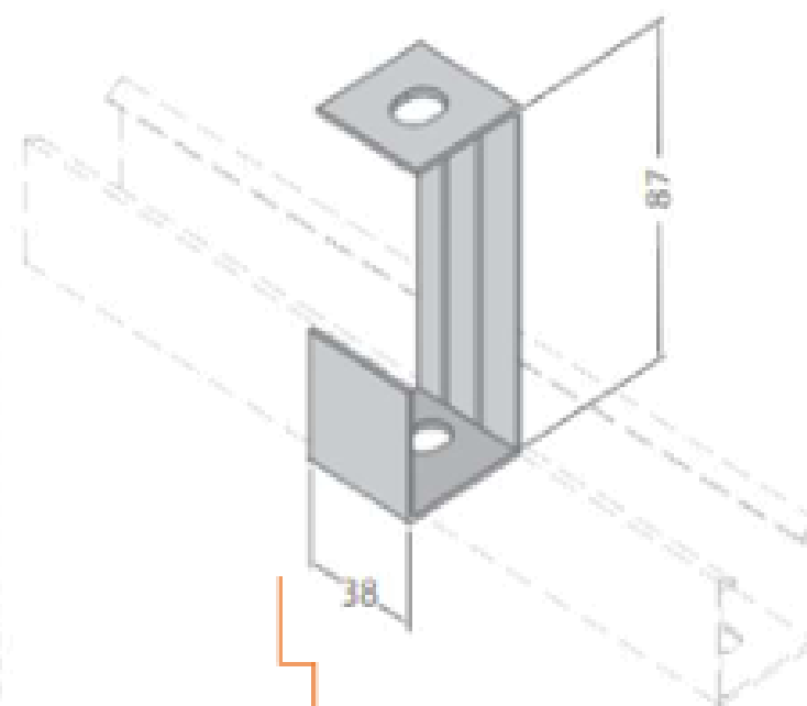
GANCHO CURTO
