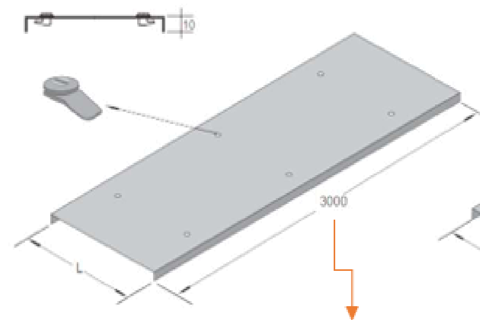
TAMP. DE ENCAIXE C/ FECHO FENDA
