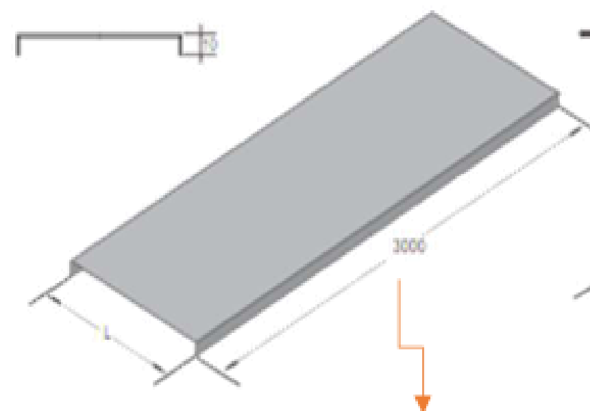
TAMP. DE ENCAIXE
