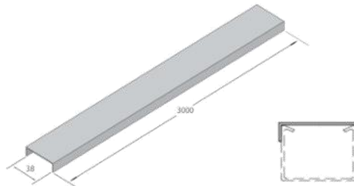
TAMPA DE ENCAIXE – 38 x 3000
