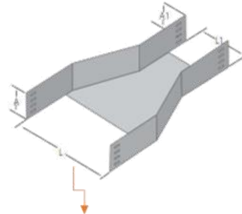
REDUÇÃO CONCÊNTRICA
