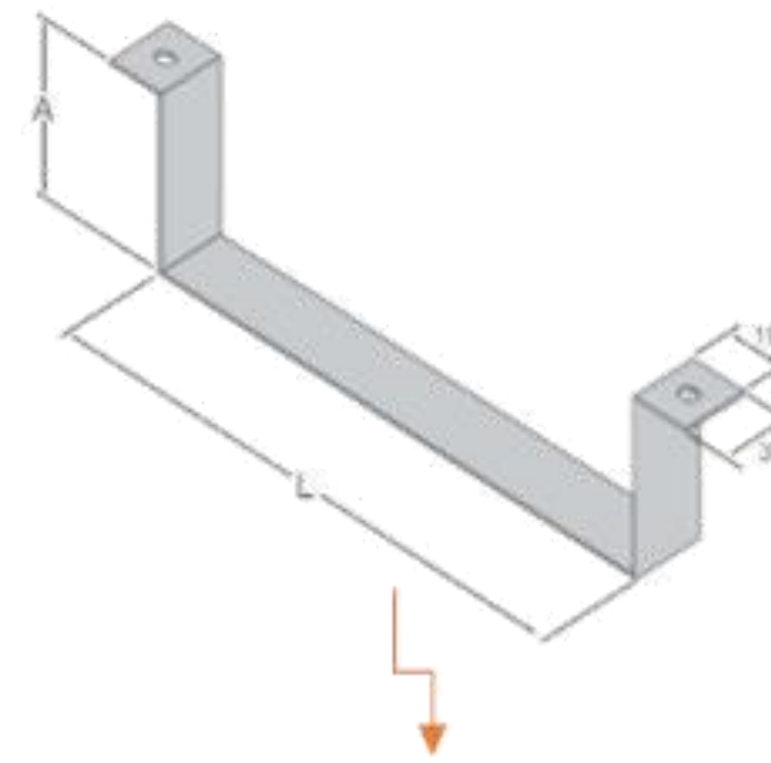
SUPORTE ÔMEGA
